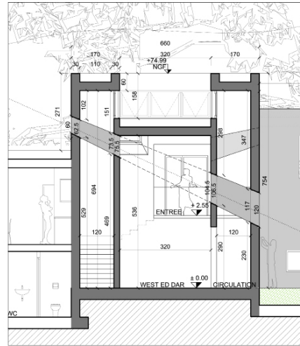
COUPE WED 2
